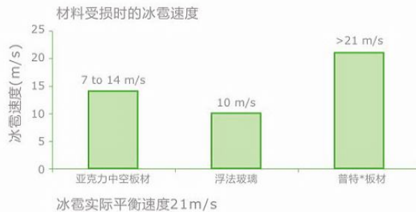
图2：耐冲击
